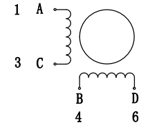
接线图 Wiring Diagram
